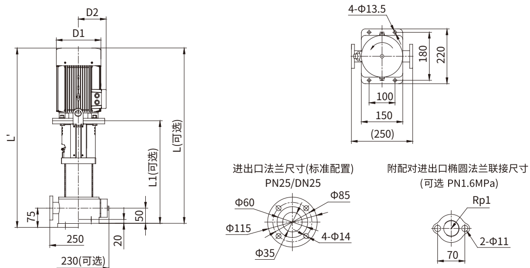
KQDP25-1G安装图
