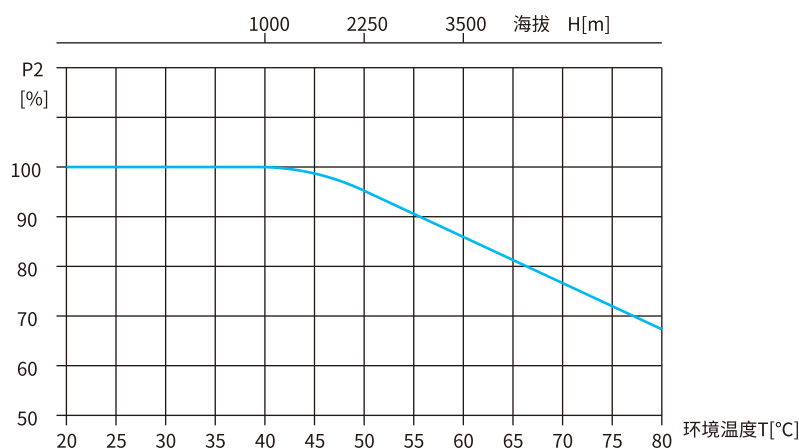
温度及海拔对电机输出功率的影响
