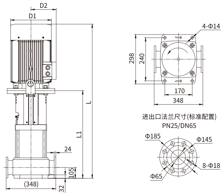
KQDQ65-32尺寸表
