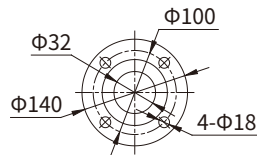
进出口法兰尺寸(标准配置) PN25/DN32
