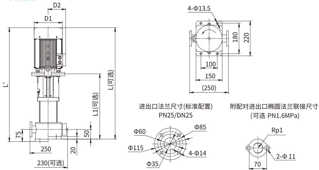
KQDP25-1安装图
