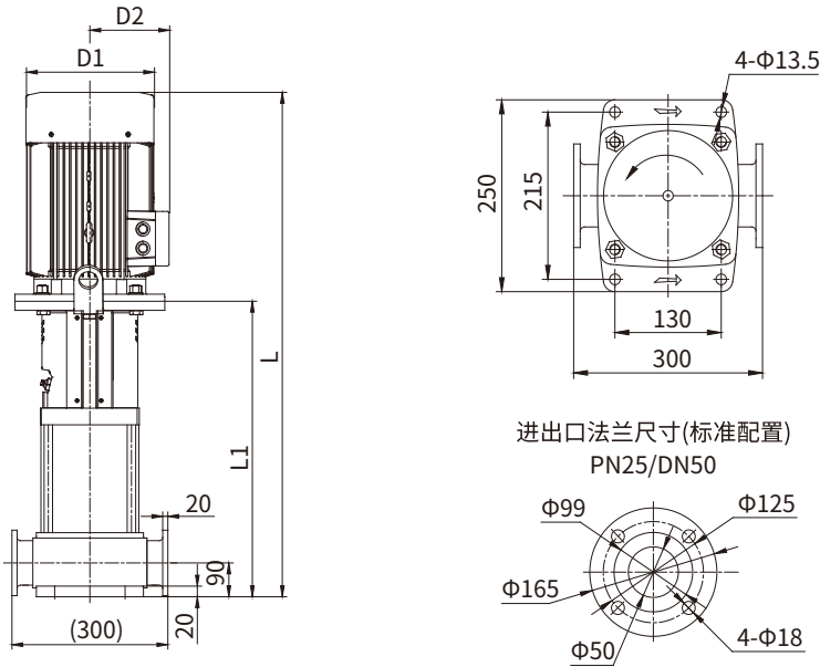
KQDP50-12安装图
