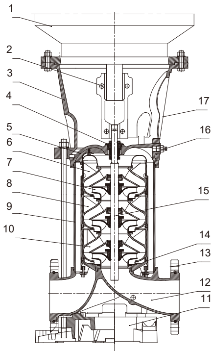
KQDQ150、125
