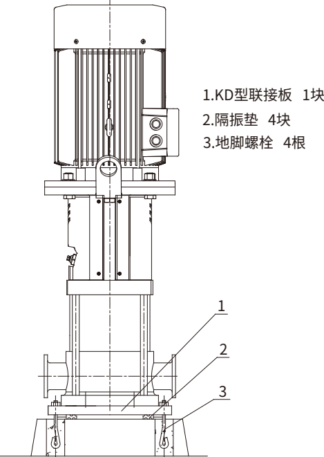
柔性连接(隔振垫)
