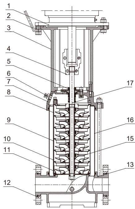
结构图 KQDP65
