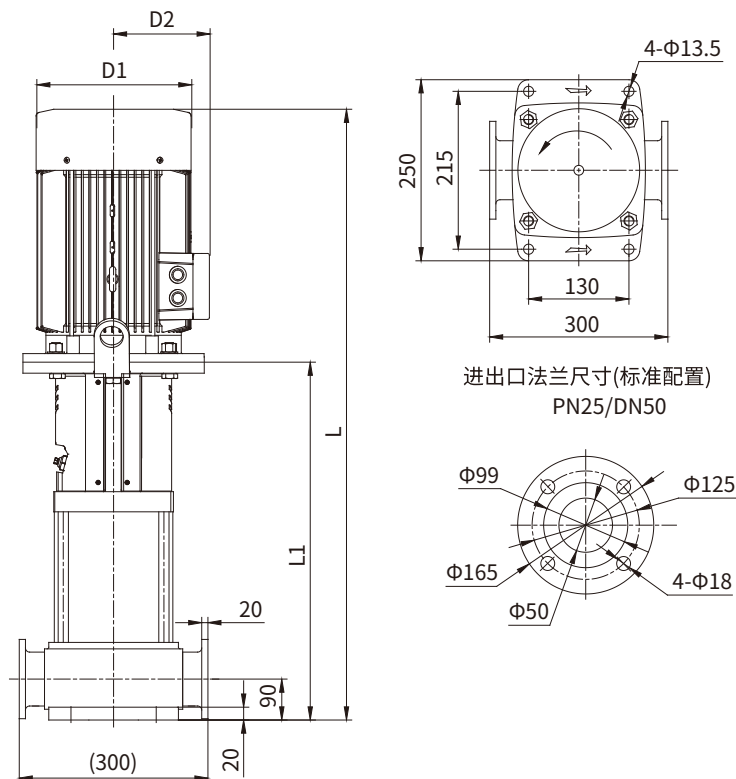
KQDP50-16安装图
