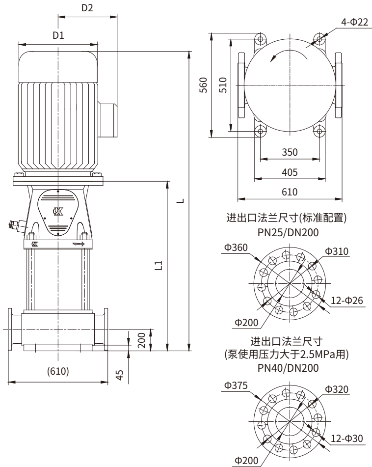
KQDP/KQDQ200-200安装图
