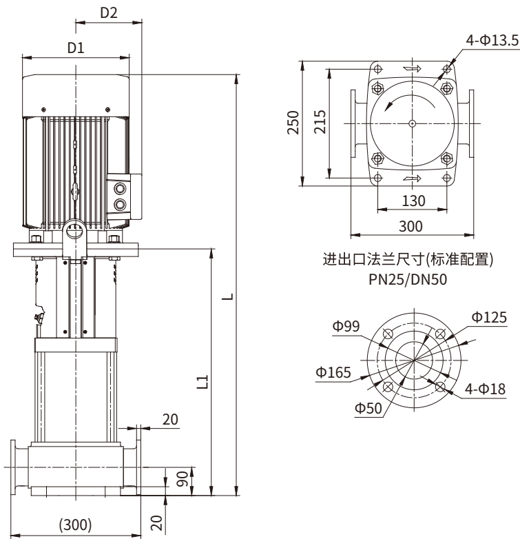
KQDP50-20安装图
