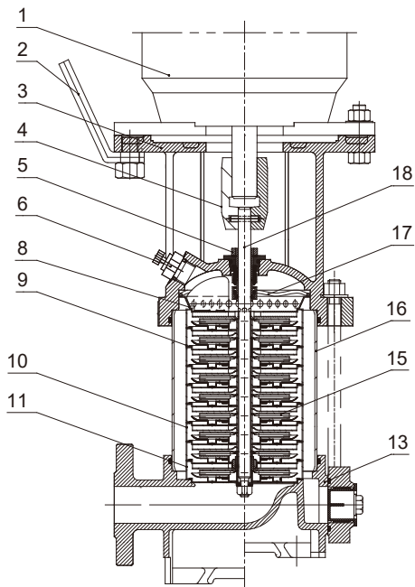
KQDQ25、32
