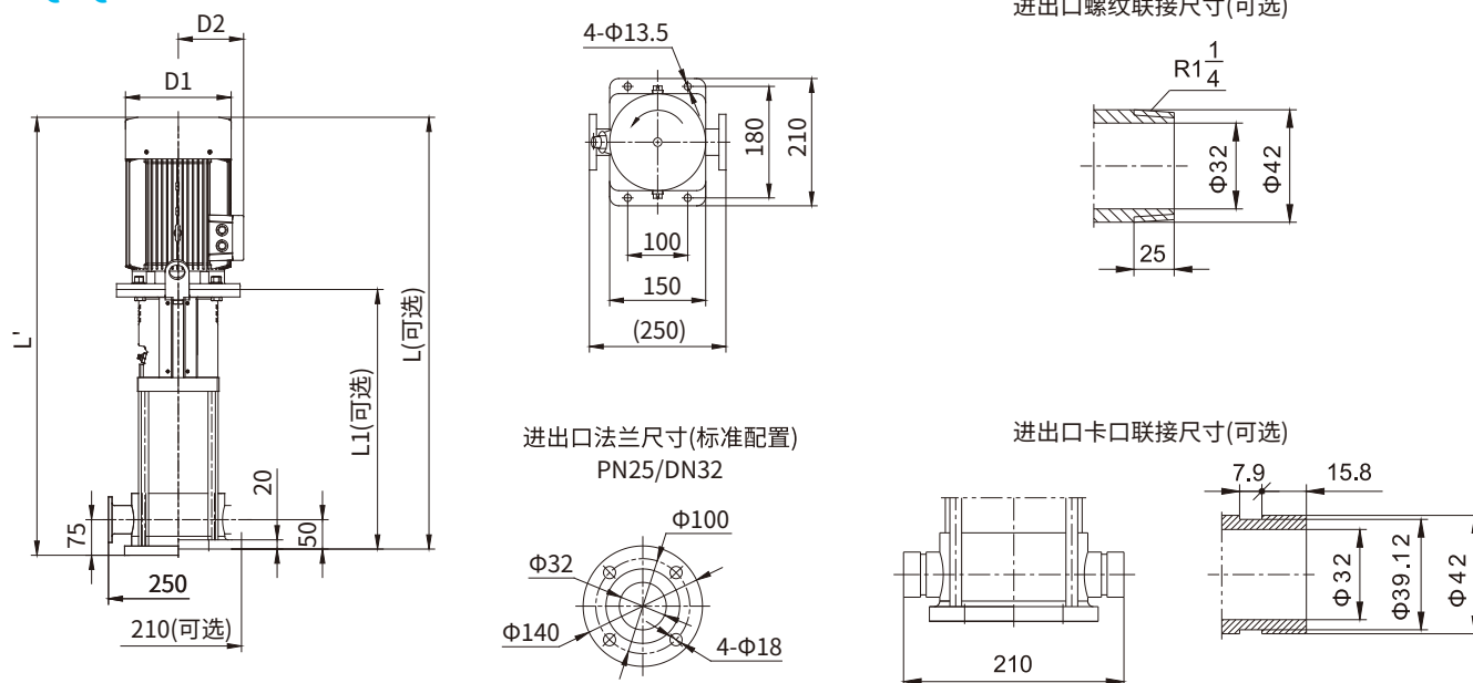
KQDQ32-4安装图
