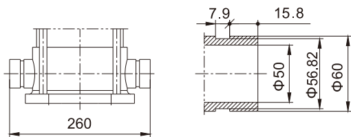
进出口卡口联接尺寸(可选)
