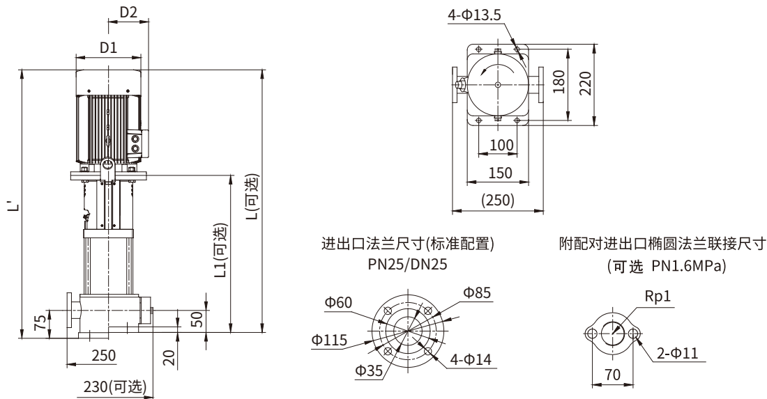
KQDP25-3安装图
