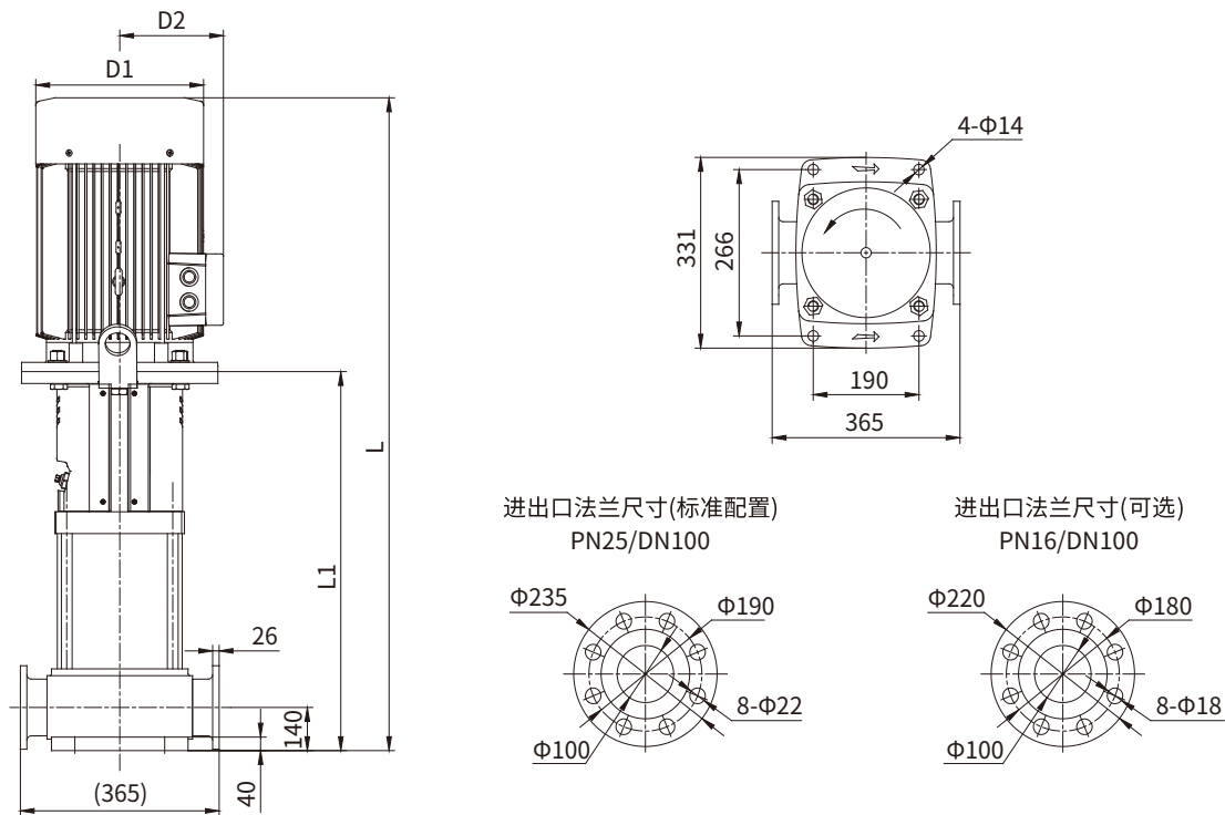
KQDP/KQDQ100-64安装图
