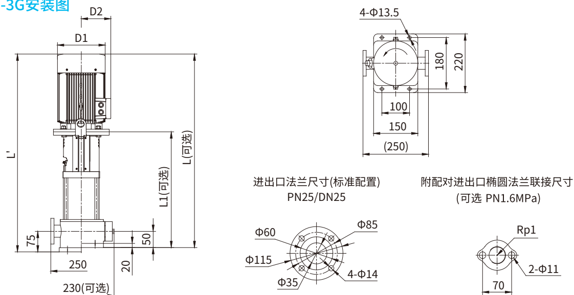
KQDP25-3G尺寸表
