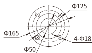
进出口法兰尺寸(标准配置) PN25/DN50
