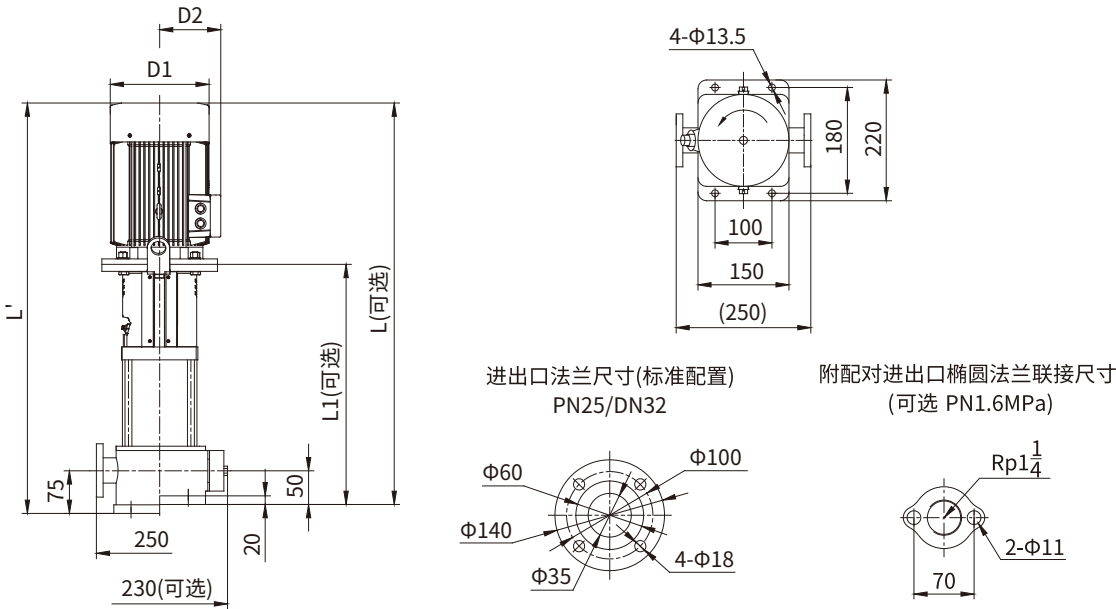
KQDP32-4安装图
