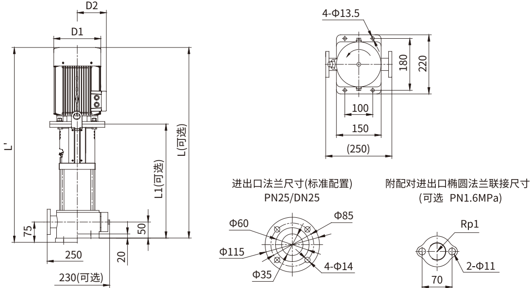
KQDP25-2安装图
