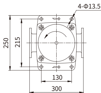
进出口法兰尺寸(标准配置) PN25/DN50
