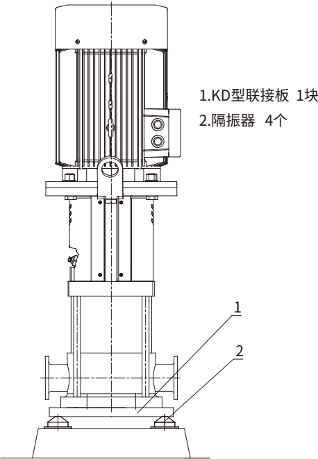
柔性连接(隔振器)
