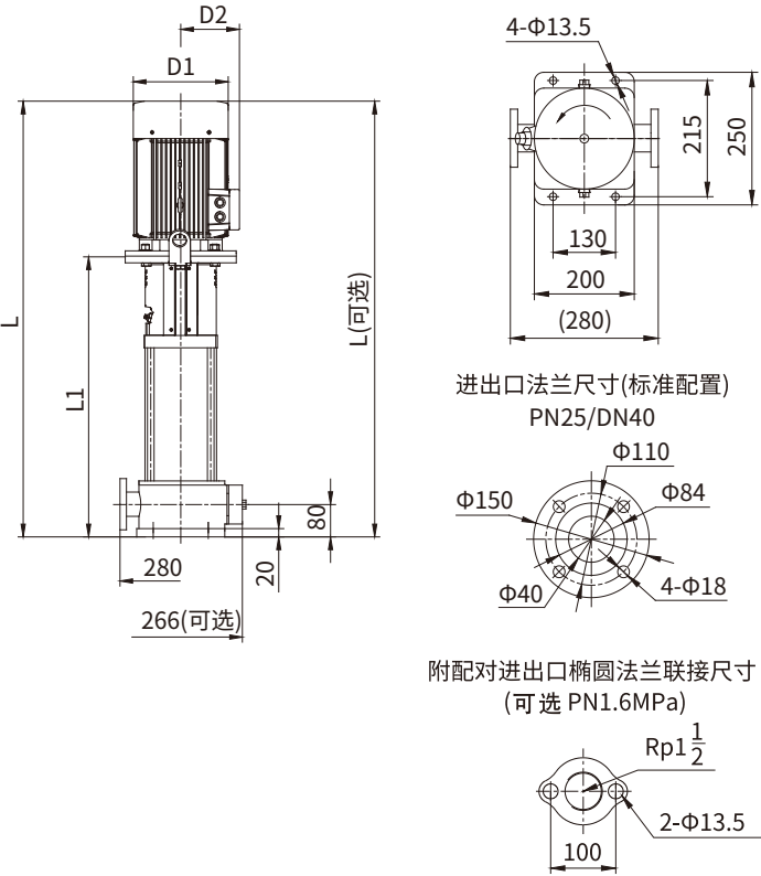
KQDP40-8安装图
