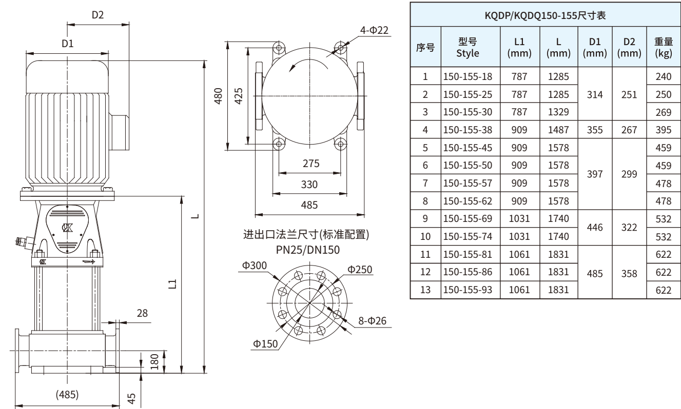
KQDP/KQDQ150-155安装图
