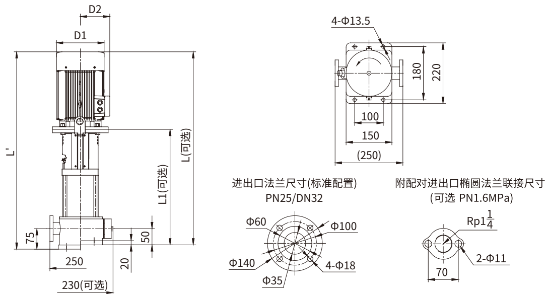
KQDP32-5安装图
