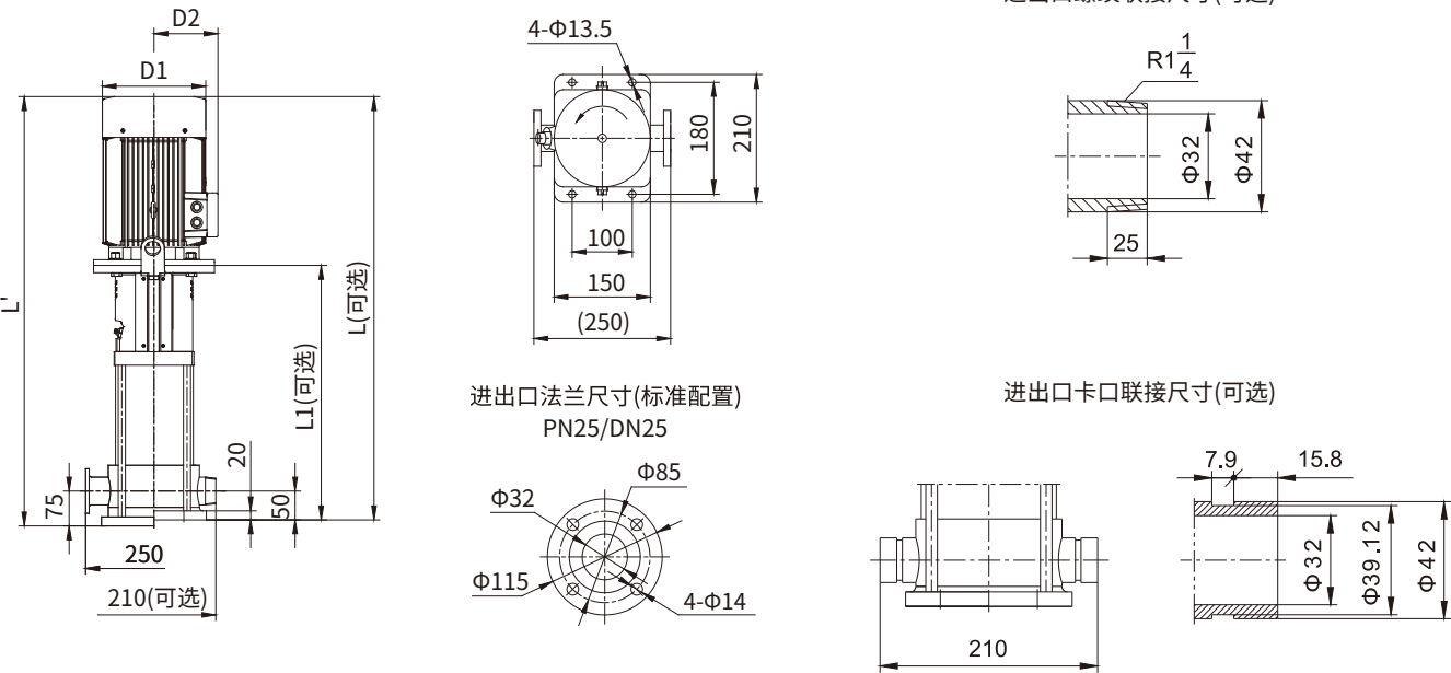
KQDQ25-1安装图
